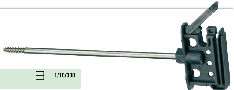
2996 AISLADOR 20 cm. ROSCA MADERA, HILOS, CINTAS, CUERDAS HASTA 40 mm.
